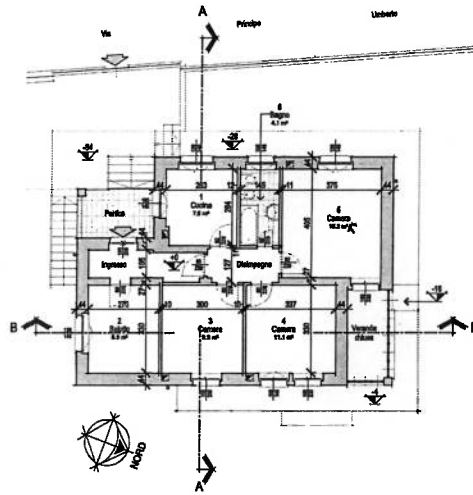
Pianta piano terreno Scale 1:100
